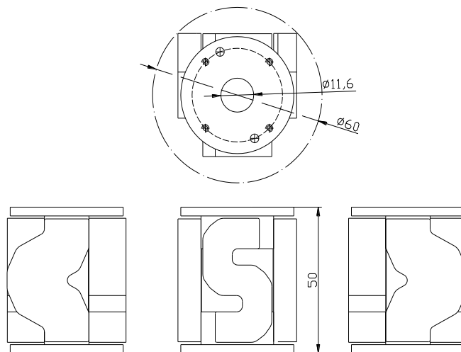
K band 180°phase shifter
